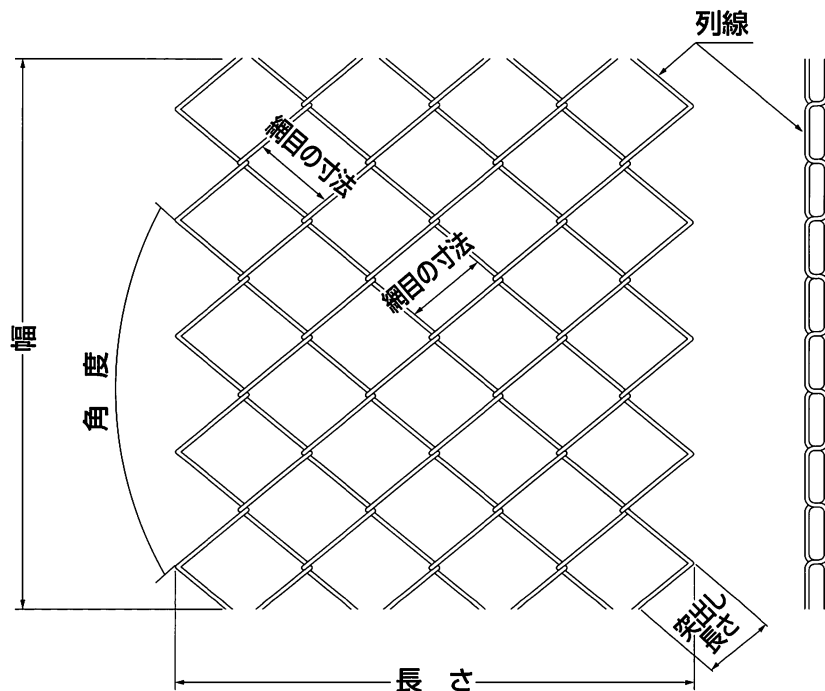
■ 図1 ひし形金網の名称
